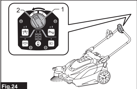
► 1. Interruptor de ENCENDIDO/APAGADO 2. Botón de desbloqueo
